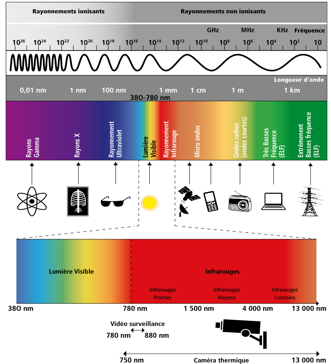
Figure 10 : Le spectre de la lumière sur l'échelle des ondes électromagnétiques.
